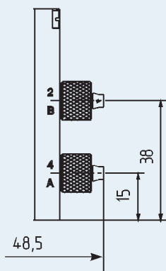
Вид 5 Под мягкую трубку 6/4 мм, спереди
