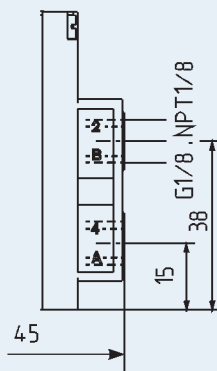
Вид 6 Резьба G 1/8, вид спереди
